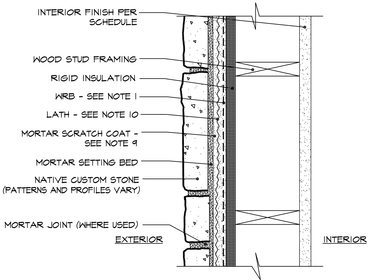
○ STONE OVER RIGID INSULATION SCALE: N.T.S.
